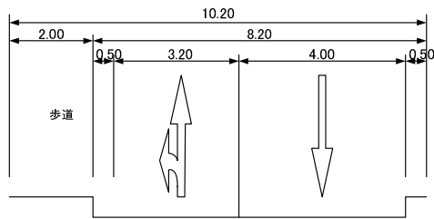
03-A断面
