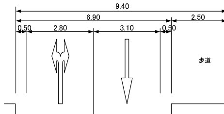
03-B断面
