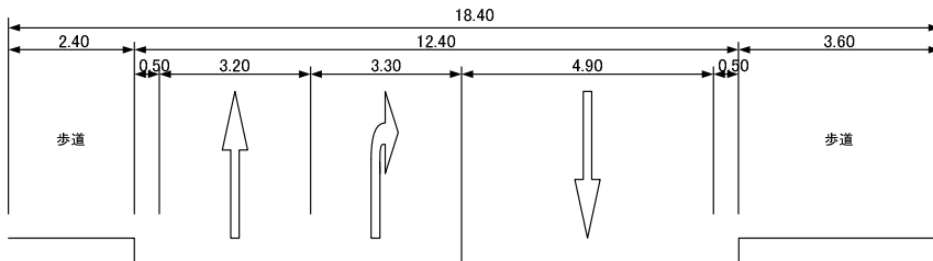
03-C断面
